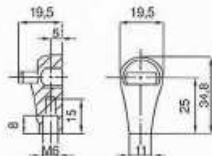
2 Cage à roulette \varnothing 10, 92720 NYLON
