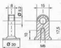
8 Chape à œil 8/8 92263 ALLIAGE
