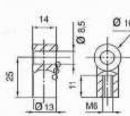
10 Chape à œil 8/14 92522 NYLON
