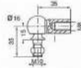
25 Cône à roulette Ø 16 92262/10-9 ACIER
