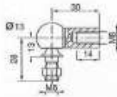
12 Cône à roulette Ø 13 92262 ACIER
