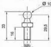
7 Roulette \varnothing 10 92990 ACIER
