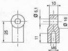
9 Chape à œil 6/10 92528 NYLON
