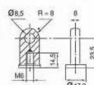
11 Chape à œil 8/8 92521 NYLON
