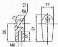
1 Cage à roulette \varnothing 10 92722 NYLON
