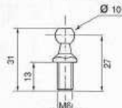
6 Roulette \varnothing 10 92989 ACIER
