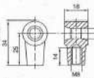
15 Coupe à roulette Ø 18 92268 ALLIAGE
